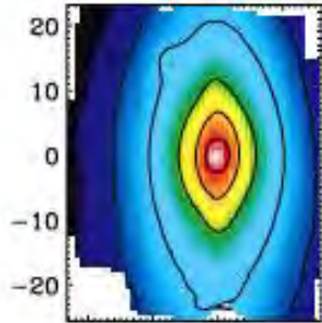
NGC 2549 ↗
