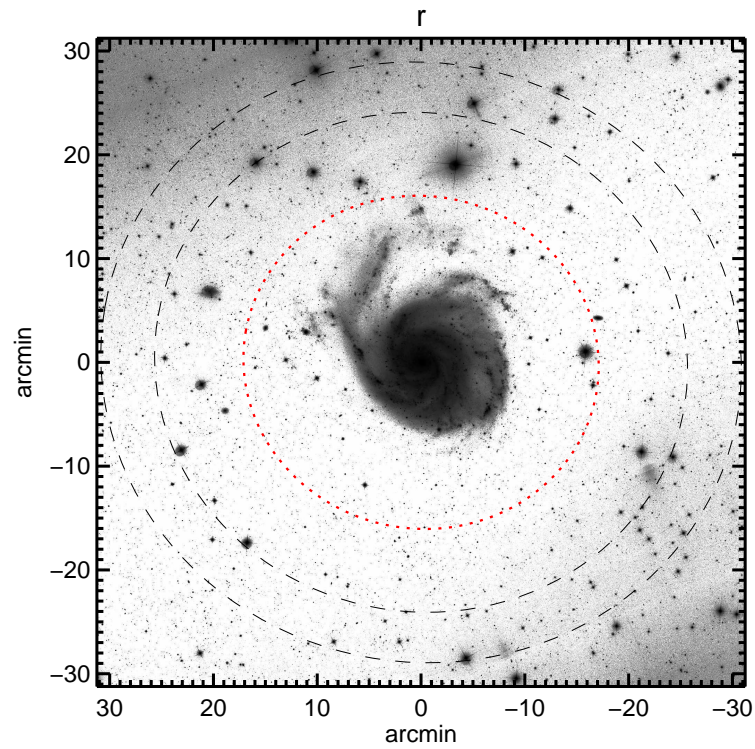
NGC5457
